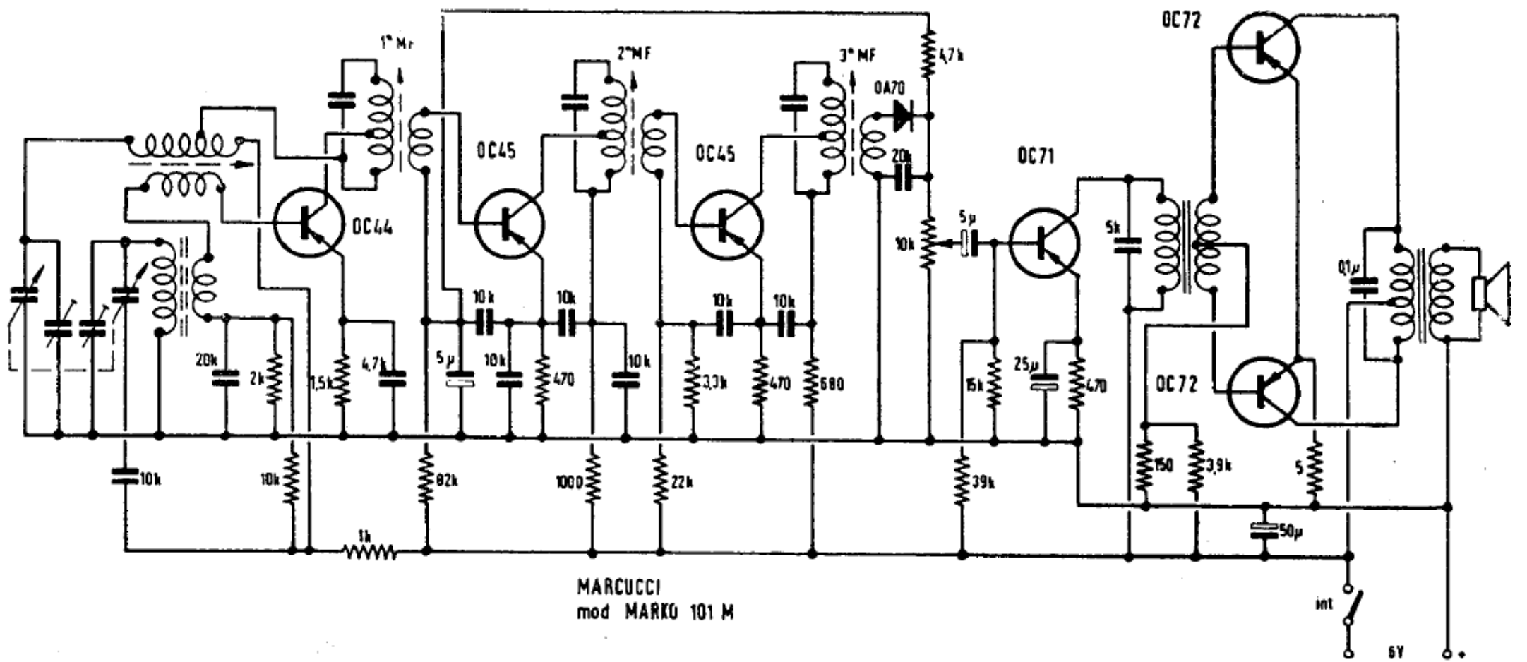
Schema elettrico del radiorecettore AM, Marcucci, mod. Marko 101 M
